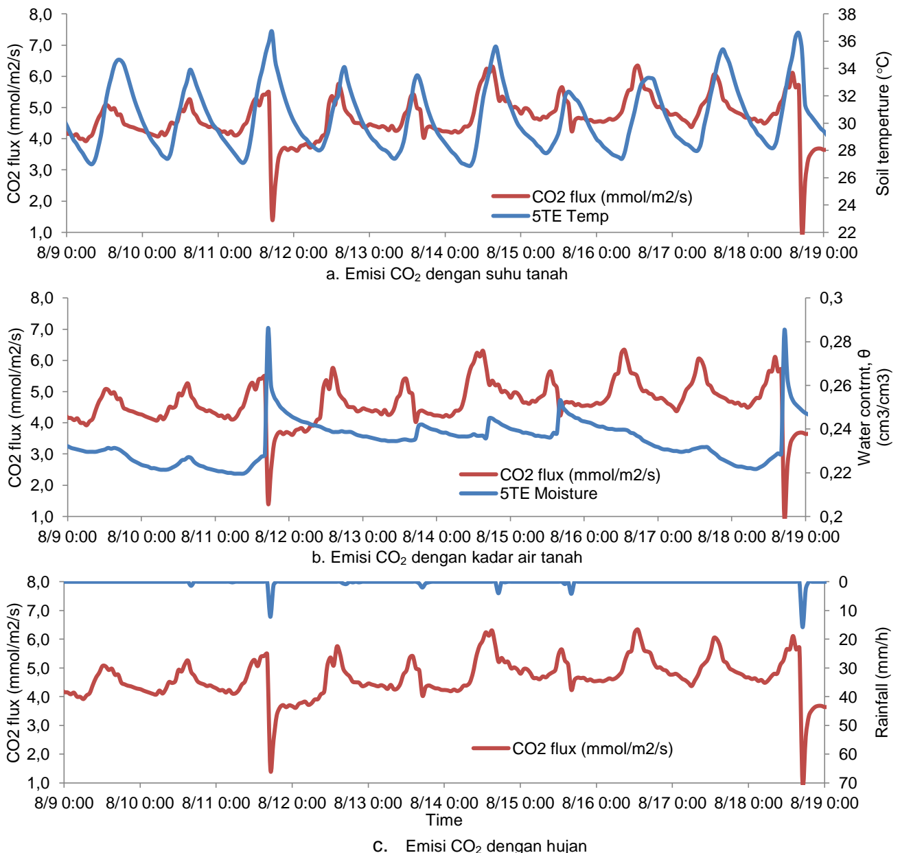
Gambar 7 Dinamika emisi CO 2 dengan temperatur tanah (a), kelembapan tanah (b), dan curah hujan (c).
