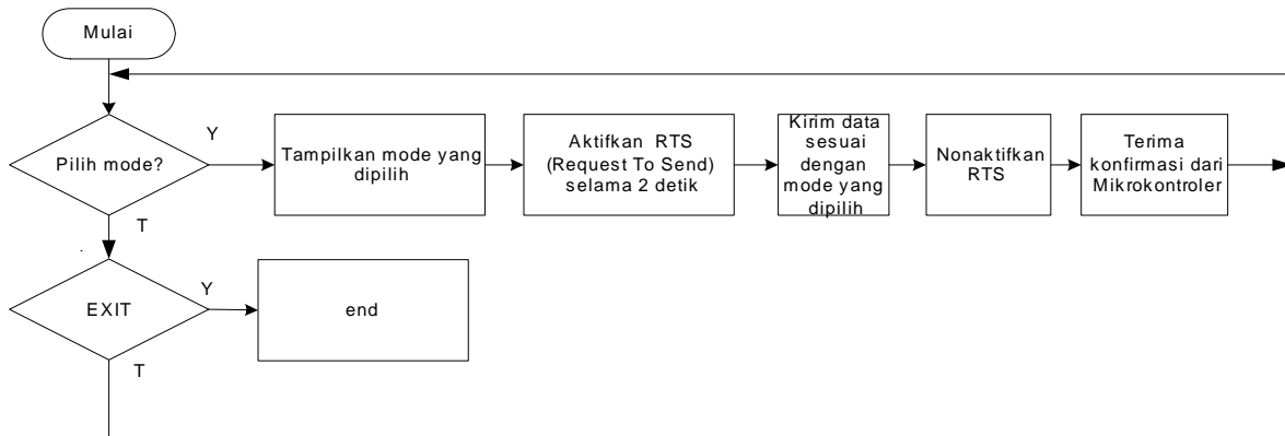
Gambar 3. Flowchart program aplikasi.
