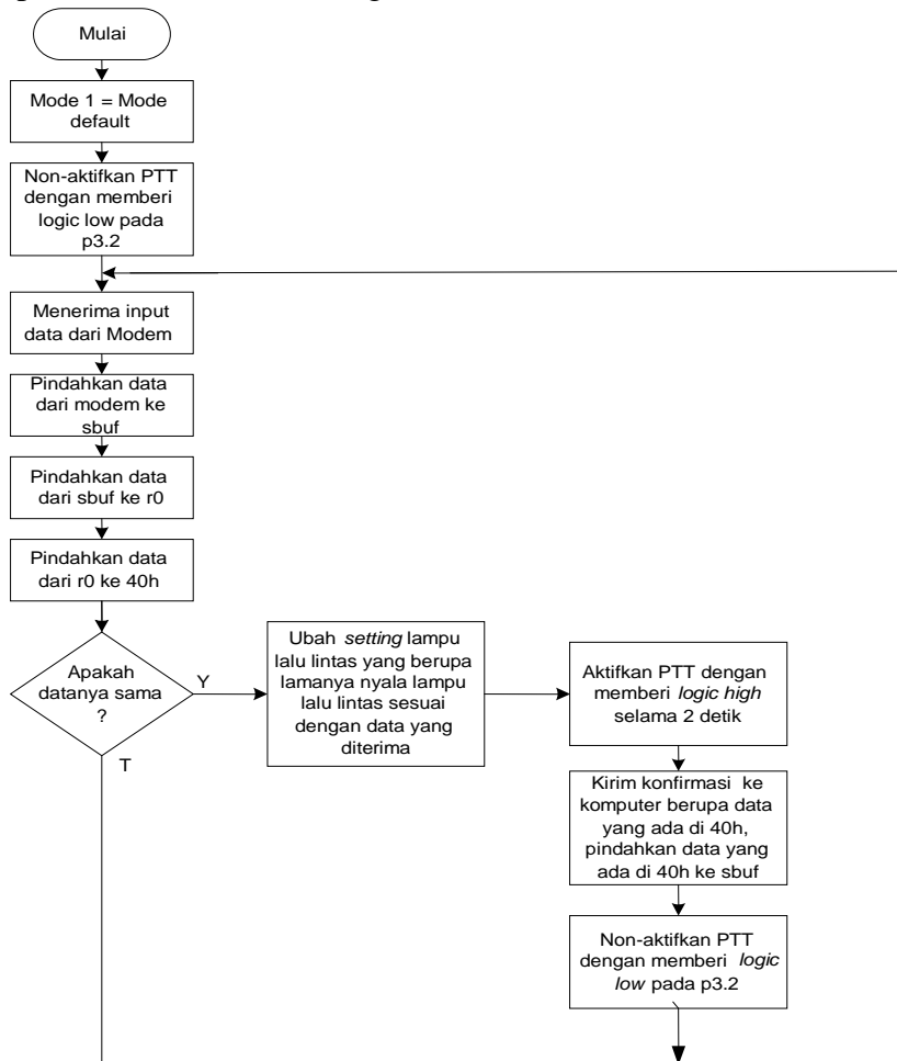
Gambar 2. Flowchart pada mikrokontroler.
