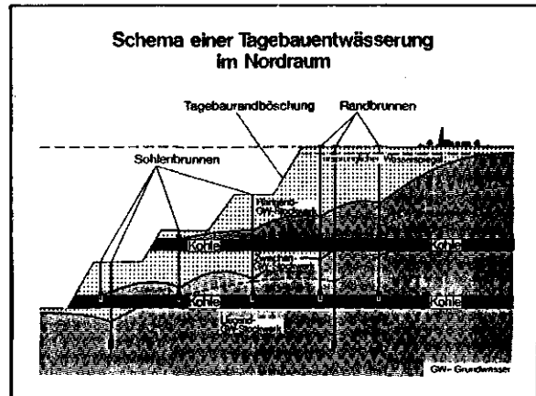
Abb. 3: Schema einer Tagebauentwässerung
