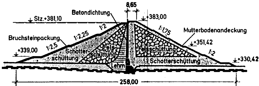
Figuur 15 Dwarsdoorsnede Söse- en Oderdam
