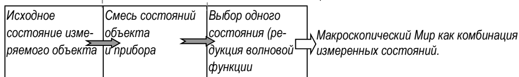
Рис. 8. Схема процесса квантового измерения.
