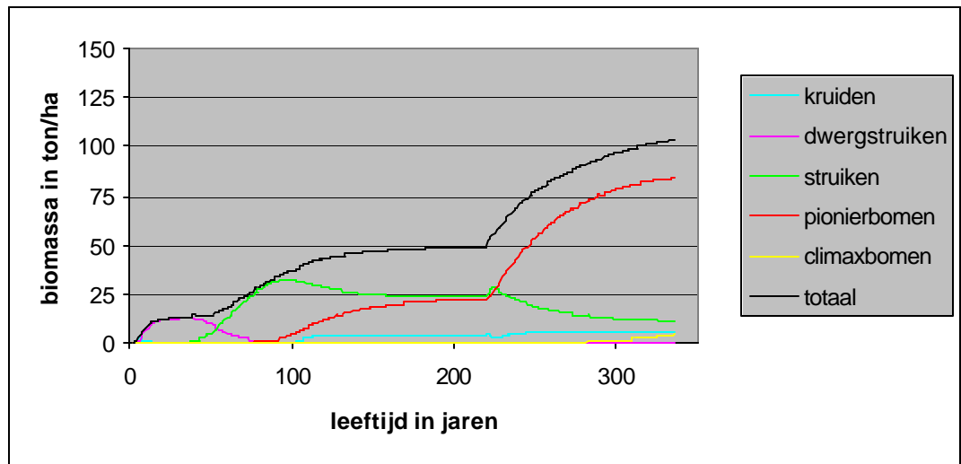
Fig. 17 Biomassaontwikkeling in het vegetatietype kaal duinzand, per functioneel type.
