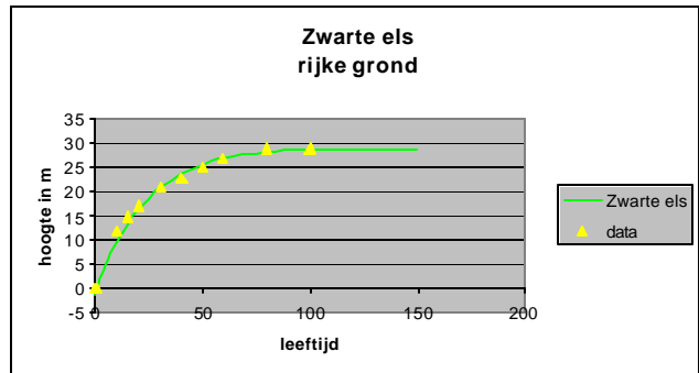
Fig. 1v. Lengtegroei van zwarte els onder voedselrijke omstandigheden; in geel de gemeten data, in groen de gefitte groeicurve. Voor uitgebreide uitleg
