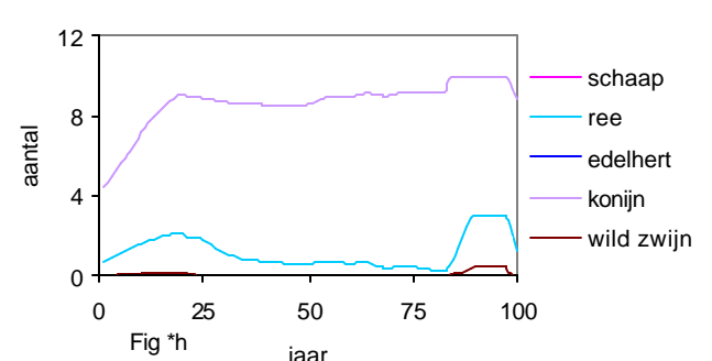
Fig. 6 a tmt i. Biomassa ontwikkeling, hoogtegroei en graasdruk op een kale grond in Zuid Limburg op kalkarme kleigrond. Fig. a geeft de biomassa ontwikkeling zonder beheer, fig. b de bijbehorende lengtegroei. Fig. c geeft de biomassa ontwikkeling met natuurlijke begrazing, fig. d de bijbehorende lengtegroei en fig. e het aantal grazers. Fig. f geeft de biomassa ontwikkeling natuurlijke begrazing en traditioneel bosbeheer, fig. g geeft de bijbehorende lengtegroei en fig. h geeft het aantal grazers.
