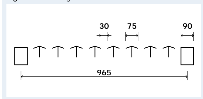
Figuur 1 Afmeting en vorm emissie-arm stalen rooster
