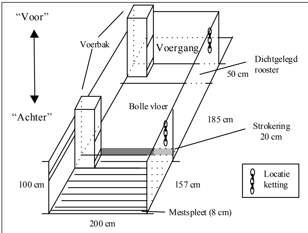
Figuur 1 Hokinrichting. Voerbak en ketting waren voor of achterin gesitueerd
