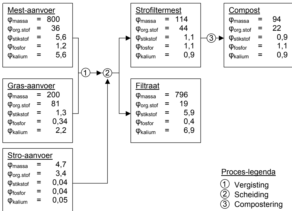
Figuur 7.2: Theoretische massabalans voor het Morveco Systeem, gebaseerd op aannames en samenstelling van de inputs. Gegevens weergegeven in tonnen per jaar.
