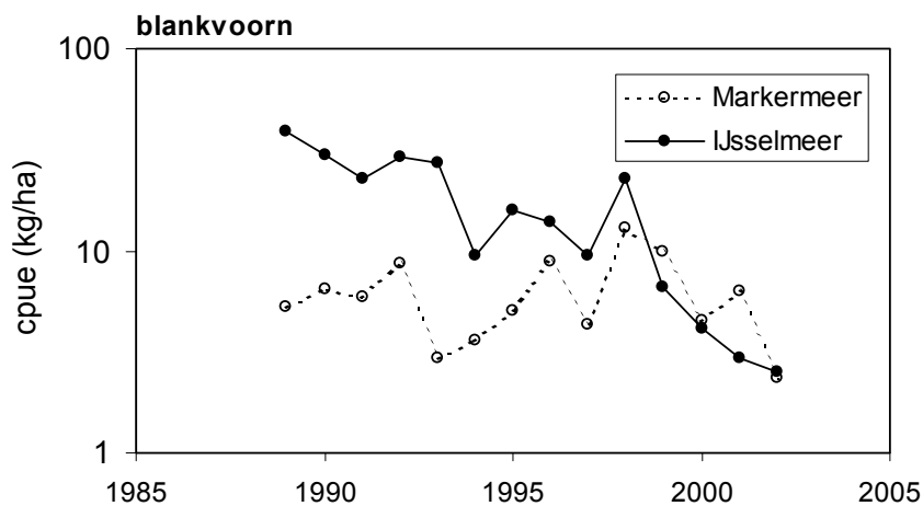
Figuur 4.5.1 Biomassa
