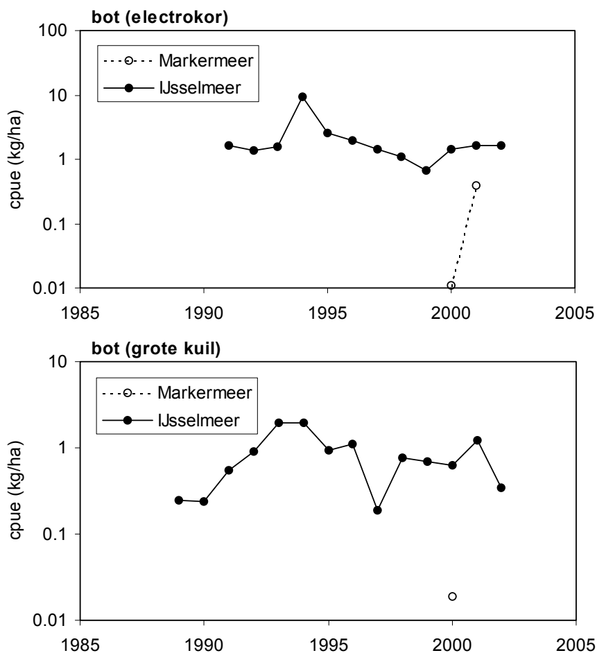
Figuur 4.7.1 Biomassa
