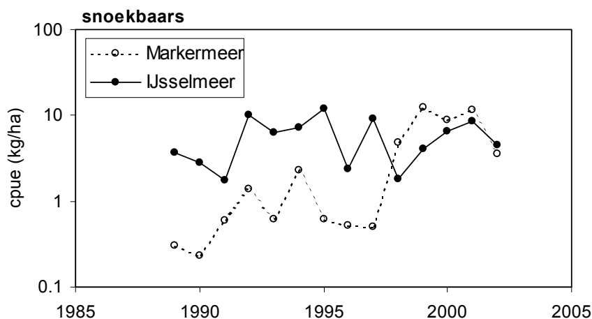
Figuur 4.2.1 Biomassa
