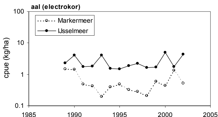
Figuur 4.1.1 Biomassa
