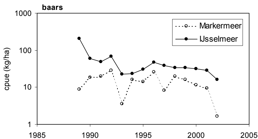
Figuur 4.3.1 Biomassa
