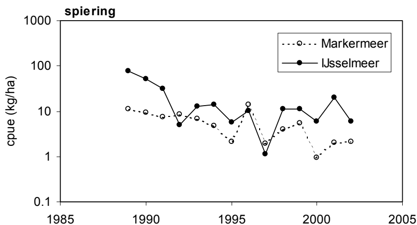
Figuur 4.4.1 Biomassa
