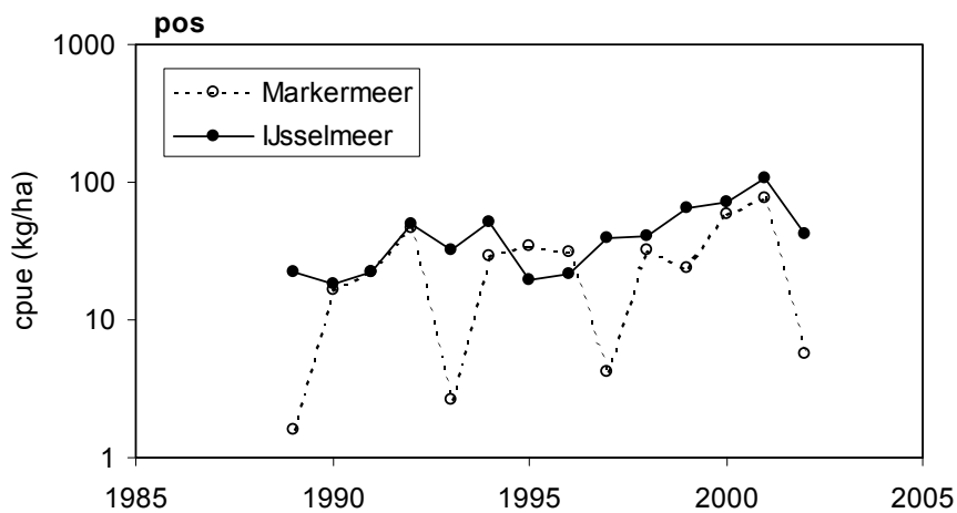
Figuur 4.8.1 Biomassa
