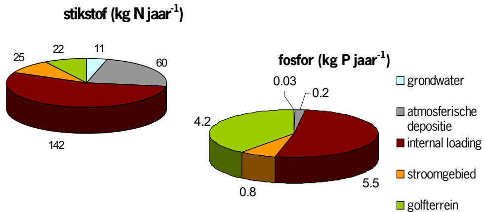
Figuur 4.30. Globale stikstof belasting (kg N jaar -1 ) (links) en de globale fosfor belasting (kg P jaar -1 ) (rechts) in de duikplas berekend over de periode augustus-november 2002.
