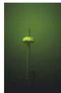
Figuur 3.3. Sedimentval (8 m diepte) in de duikplas.
