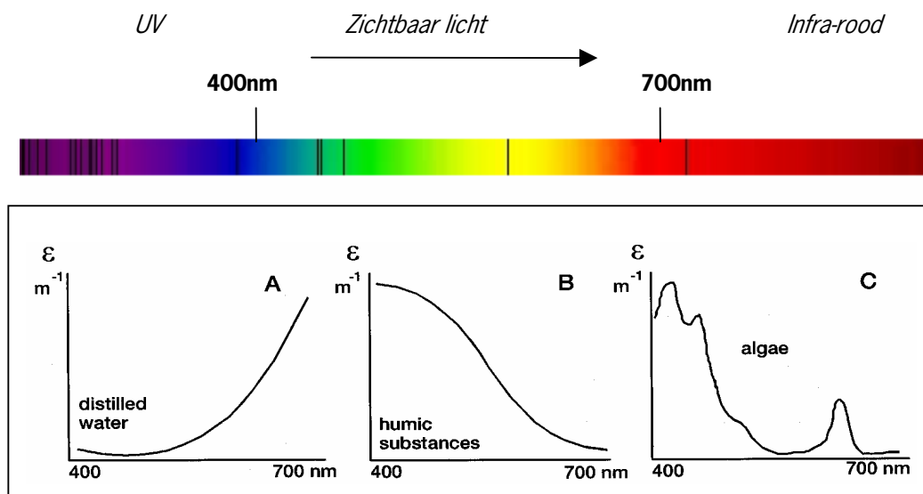
Figuur 2.4. Lichtspectrum met een indicatie van de photosynthetische actieve radiatie (boven) en absorptiecurven (onder) voor A. gedistilleerd water, B. Humuszuren en C. algen.
