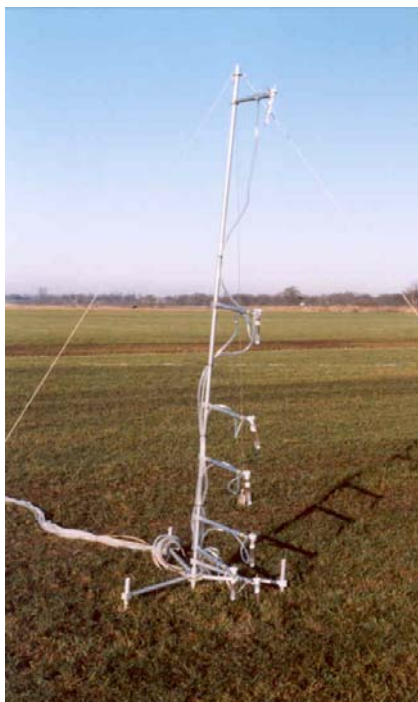
Centrale meetmast met 7 meetpunten met daarnaast één meetpunt (een gaswasfles met absorptievloeistof met impinger).
