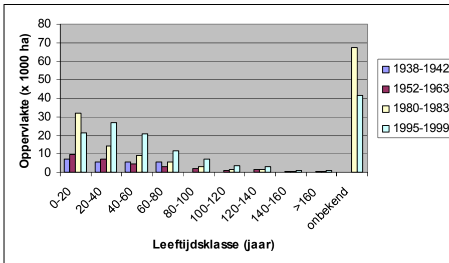
Figuur 26. Leeftijdsklassenverdeling van alle loofboomsorten in respectievelijk de eerste, tweede, vierde bosstatistiek en volgens de EFSOS data
