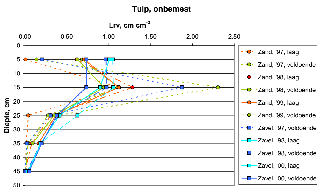
Figuur 3. Wortellengtedichtheden van tulp op zand en zavel in 1997, 1998, 1999 (zand) en 2000 (zavel) in de bodemlagen 0-10 cm, 10-20 cm, 20-30 cm en 30-40 cm bij lage en voldoende fosfaattoestand zonder fosfaatbemesting, gemiddeld over de 1 e en 2 e positie in het horizontale vlak.
