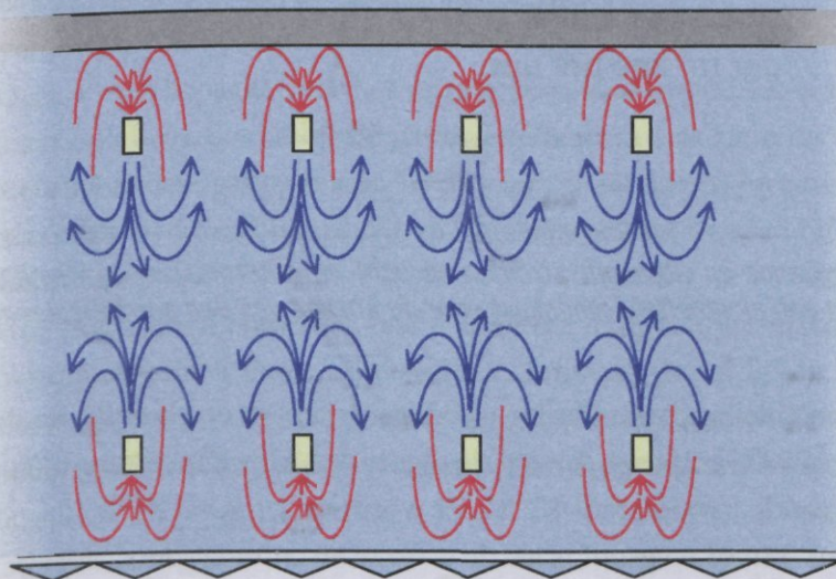
Figuur 3-2 Bovenaanzicht koelsystemen op basis van koelunits met een vrije uitblaas. Dit soort systemen wordt gebruikt bij teelten zoals phalenopsys en fresia .
