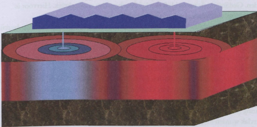
Figuur 5-2 Schets van een kas waaronder het watervoerende zandpakket wordt gebruikt voor de seizoensopslag van warmte
