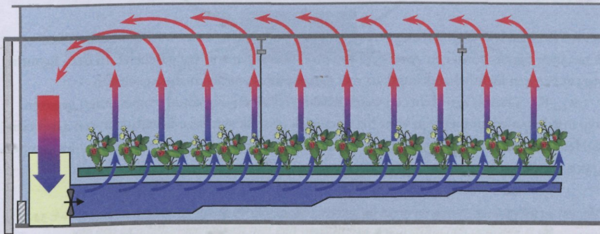
Figuur 3-1 Zijaanzicht van het luchtcirculatiesysteem, vergelijkbaar met het systeem dat beproefd wordt bij themato
