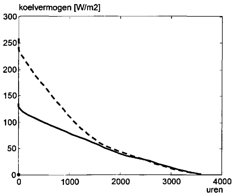
Figuur 4-5 Jaarbelastingduurkrommen van het benodigde koelvermogen voor de installatie met de kleine capaciteit (getrokken lijn) en met de grote capaciteit (onderbroken lijn).
