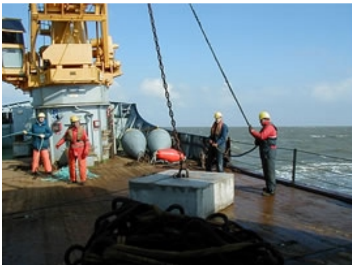
Figuur 5. Anker stenen voor longlines. www.awi-bremerhaven.de
