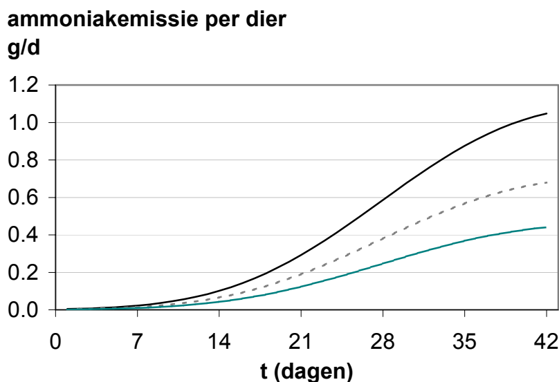
Figuur 3.3 Relatie tussen leeftijd (t, in dagen) en ammoniakemissie voor een vleeskuiken bij een constante, gemiddelde temperatuur van 5°C (onderste curve), 15 °C (middelste curve) en 25 °C (bovenste curve). De curves zijn gebaseerd op een dataset van de stalmeetploeg bij huisvesting in een traditionele stal.
