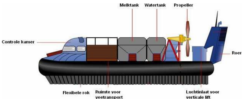
Figuur 17 Hovercraft
