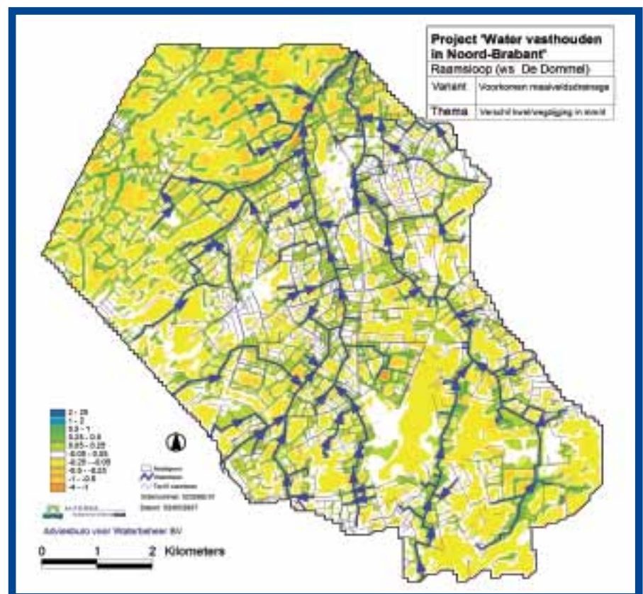
Afb. 9: Verandering van het kwelpatroon als gevolg van het 'blokkeren van de maaiveldafvoer' in het voorbeeldgebied Raamsloop.
