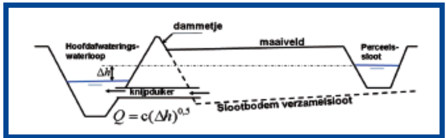
Afb. 3: Situatieschets van een knijpduiker.
