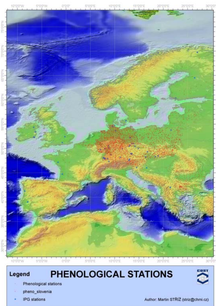
Abbildung 2: Phänologische Beobachtungsstationen
