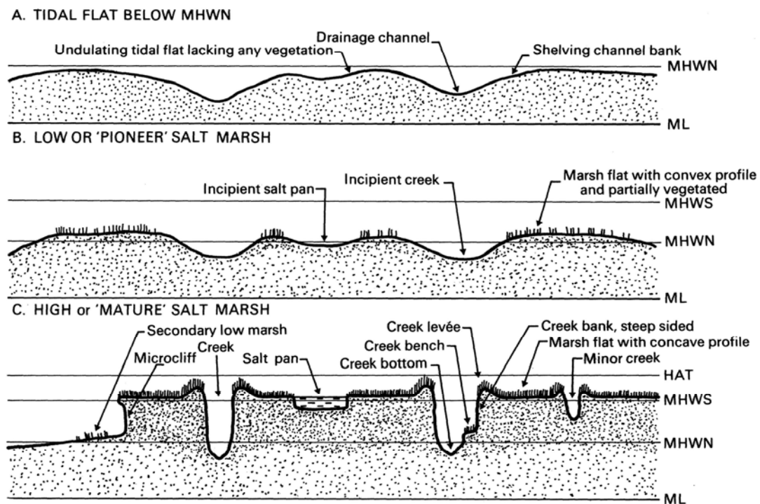
Figuur 2.3 Vorming van patronen van krekens, oeverwallen, kommen, plassen en kliffen in een kwelder (Long & Mason 1983).
