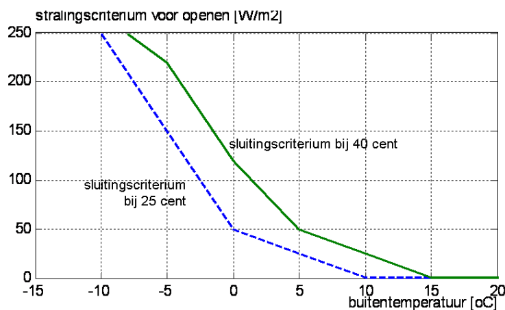
Figuur 6. Gebruikte relatie tussen het stralingscriterium waarboven het scherm 's ochtends open loopt en de op dat moment geldende buitentemperatuur. De doorgetrokken lijn is het resultaat van optimalisaties bij een gasprijs van 40 cent per \text{m}^3 . De blauwe, onderbroken lijn is een curve die is geoptimaliseerd bij een gasprijs van 25 cent per \text{m}^3 .
