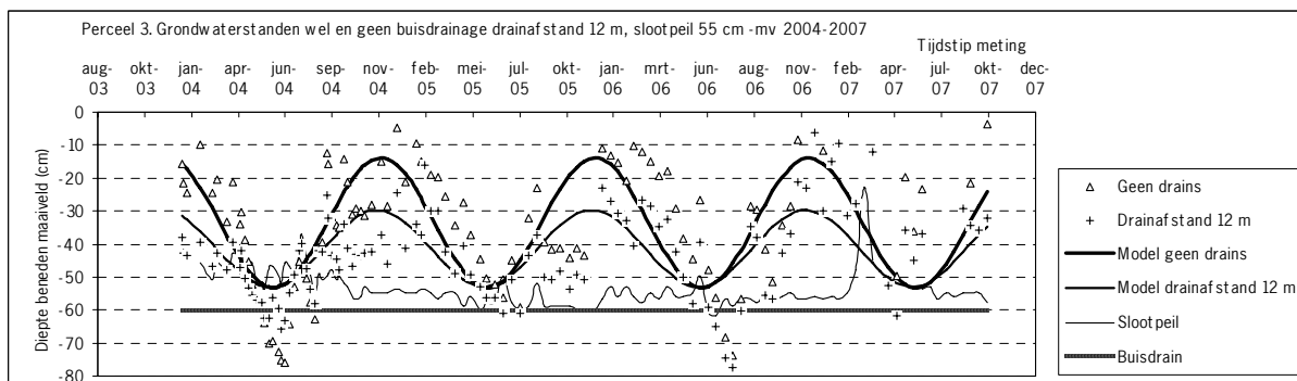
Figuur 10 Gemodelleerde en werkelijke grondwaterstanden wel en geen buisdrainage (12 m) midden perceel 3
