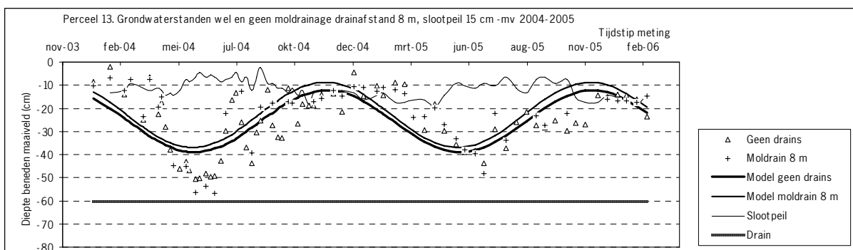
Figuur 8 Gemodelleerde en werkelijke grondwaterstanden wel en geen moldrainage (8 m) midden perceel 13
