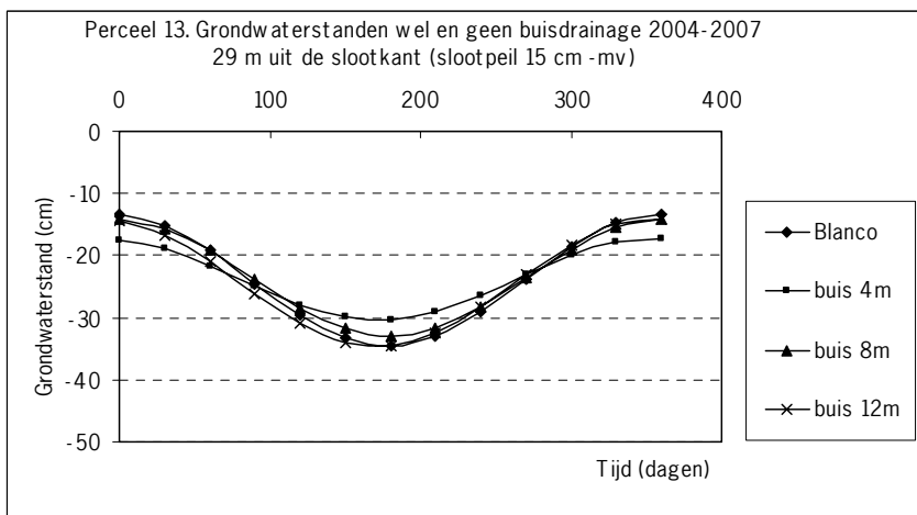
Figuur 12 Gemodelleerde grondwaterstanden wel en geen buisdrainage perceel 13, drainafstanden 4, 8 en 12 m, afstand tot de slootkant 29 m
