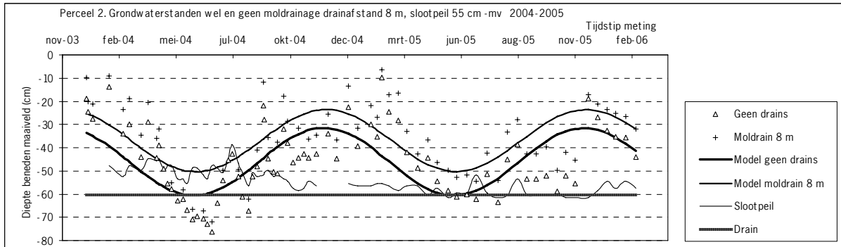
Figuur 5 Gemodelleerde en werkelijke grondwaterstanden wel en geen moldrainage (8 m) midden perceel 2
