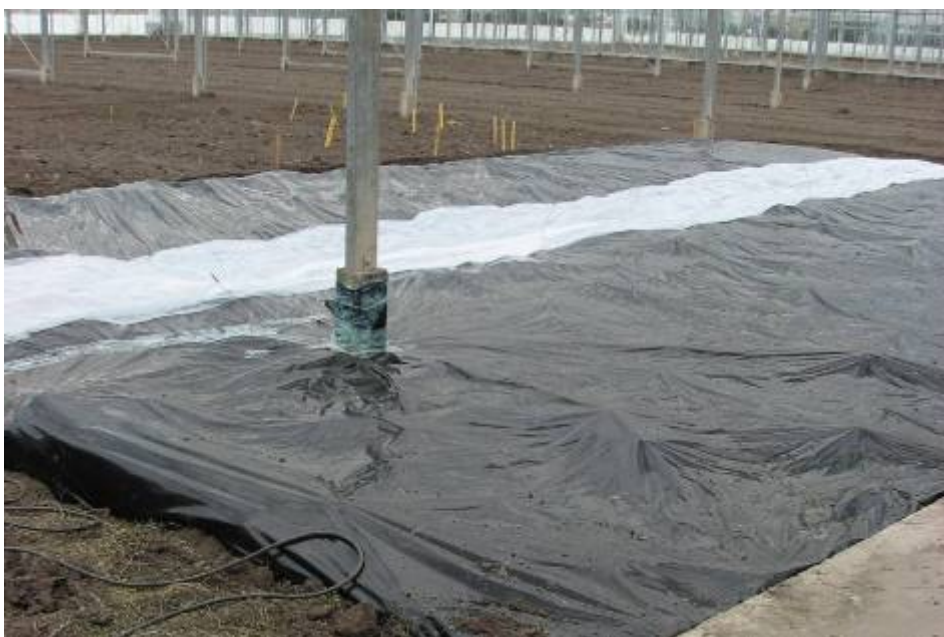
Figuur 8. Proefvak met biologische grondontsmetting in praktijkkas
