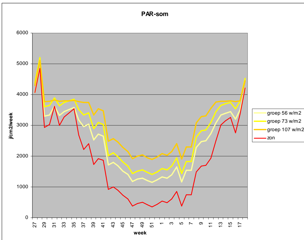
Figuur 3. PAR-som in de kas van zon en belichting van drie groepen
