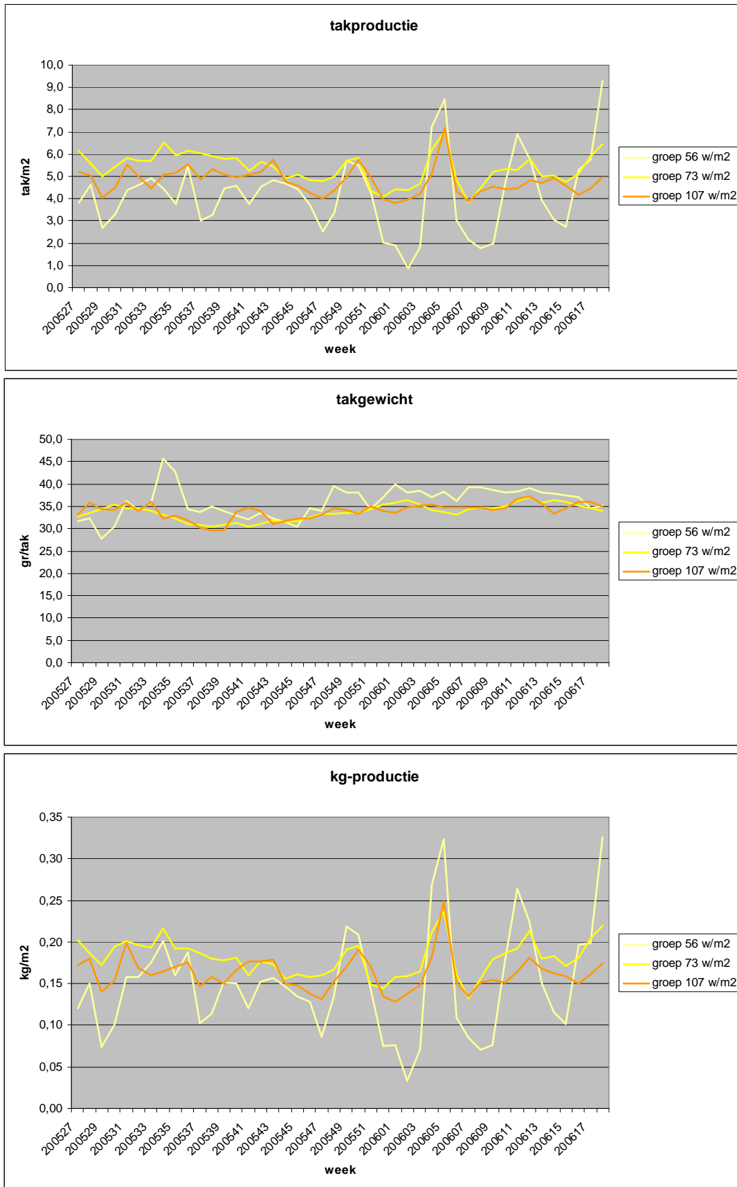
Figuur 2. Verloop van takproductie, takgewicht en kg-productie van drie belichtingsniveaus
