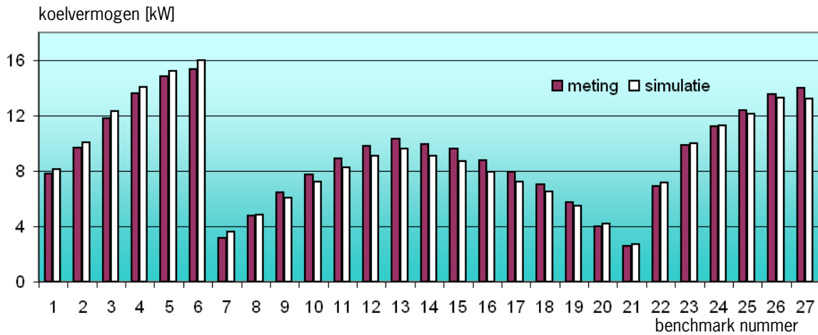
Figuur 12. Vergelijking van metingen en simulatie van de FiWiHex warmtewisselaar
