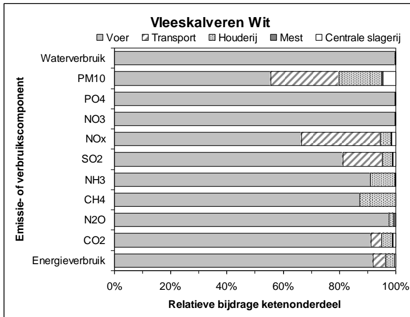
Figuur 3.2 Relatieve bijdragen van de vijf ketenonderdelen aan de totale emissies en verbruiken in de witvleeskalverproductieketen, weergegeven per emissie- of verbruikscategorie
