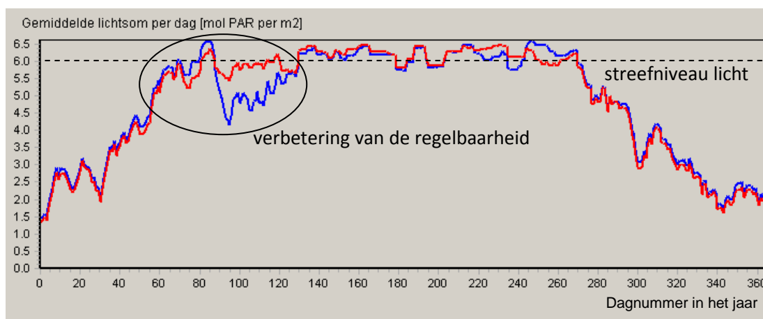
Figuur 4. Verloop van de lichtsom in een kas waar het krijt vervangen is door een extra scherm (met dezelfde schaduwfactor als het krijt) (rode lijn). De blauwe lijn is een kopie van de vorige figuur.
