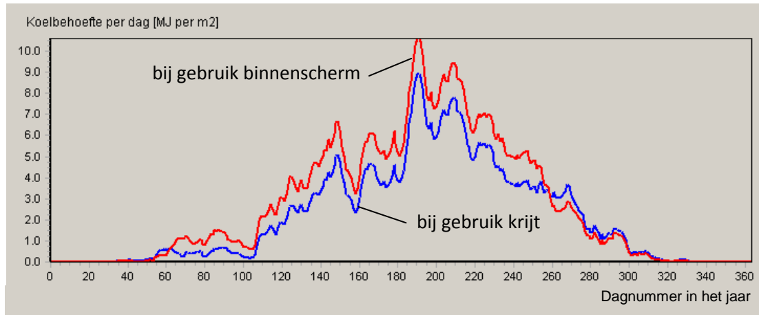
Figuur 5. Effect van de toepassing van een regelbaar binnenscherm in plaats van krijt op de koellast van een op 6 mol per m 2 per dag geschermd teelt op de benodigde koelenergie per dag bij een teelt die op 18 °C wordt gehouden. Het gebruik van een regelbaar binnenscherm leidt tot 200 MJ per m 2 per jaar extra koelbehoefte ten opzicht van het gebruik van krijt (maar geeft 5% meer licht per jaar voor de plantengroei).
