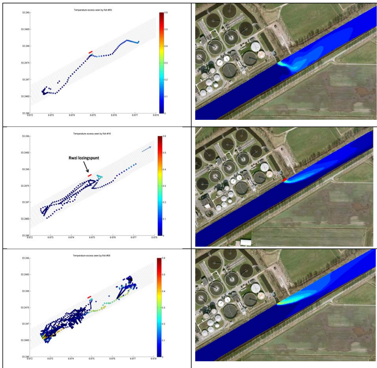
Figuur 8 Voorbeelden van zwemgedrag van schieralen bij benadering van de lozingspluim uit rwzi Garmerwolde in het Eemskanaal. In de linkerkolom is de positie van de vis in het kanaal weergegeven (blauwe stippen) ten opzichte van het lozingspunt (rode streepje) en watertemperatuur (als maat voor de effluentconcentratie) waarin het dier zich bevond zoals uitgerekend op basis van het gemodelleerde gedrag van de pluim. In de rechterkolom is de gemodelleerde invloedsfeer van de lozingspluim weergegeven op het moment dat de vis de rwzi passeert.
