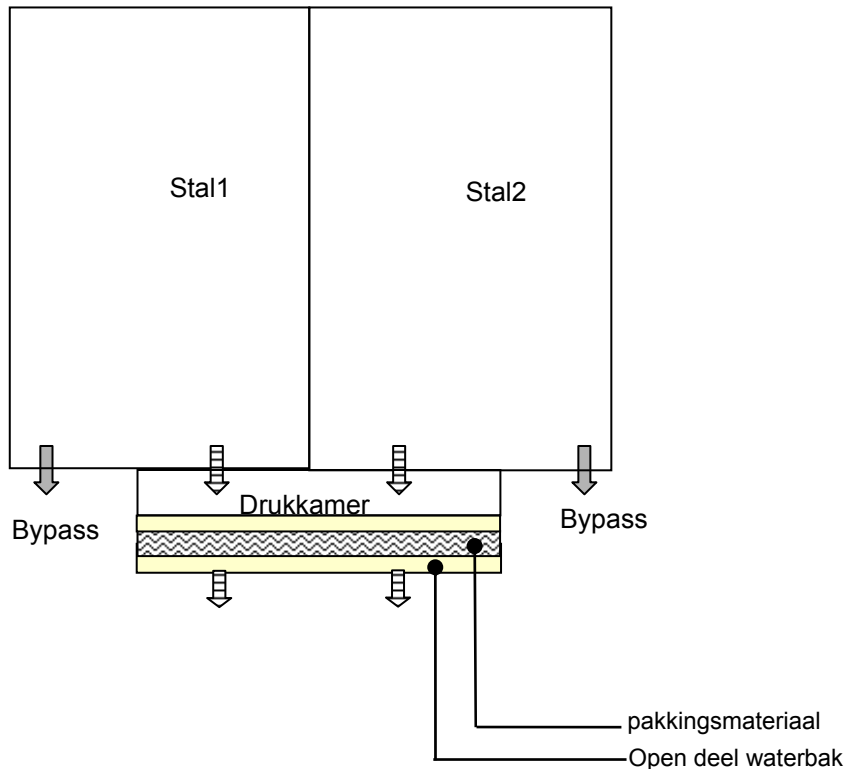
Figuur 2 Bovenaanzicht waterwasser bedrijf 2 met daarin de luchtstroming door de waterwasser (gestreepte pijlen), en door de bypass (grijze pijlen)
