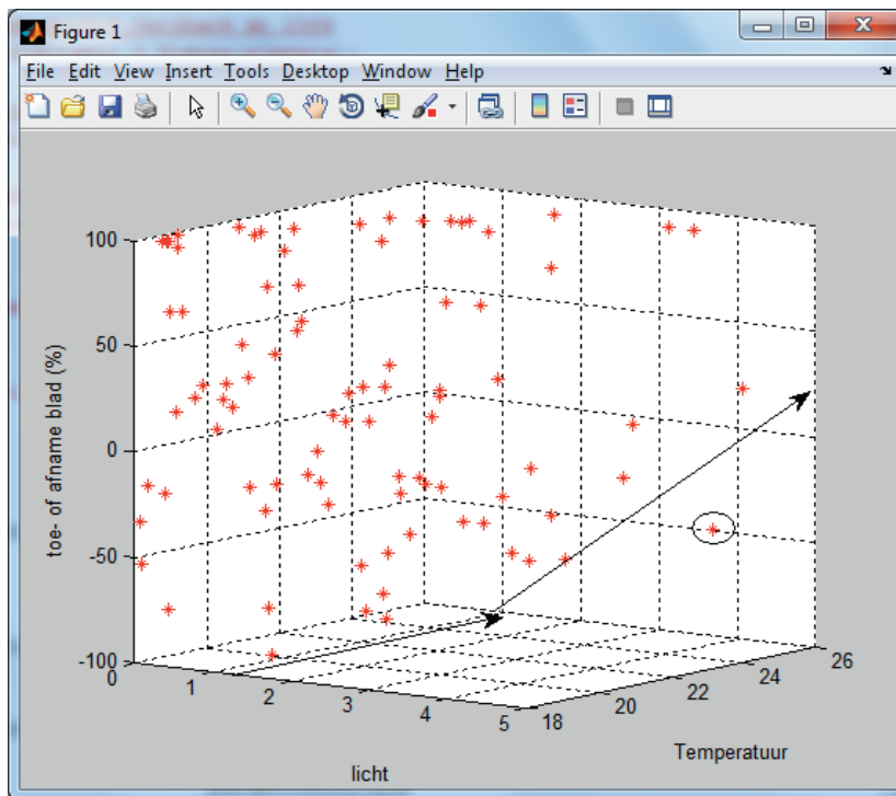
Figuur 3.9. De effecten van licht (MJ PAR/m 2 /d) en etmaaltemperatuur (°C) op de toename of afname van het bladoppervlak per gewaslaag van 5 internodia, uitgezet in een 3D grafiek. Elk sterretje geeft een resultaat aan van een tijdvak tussen twee oogsten. Data van alle bedrijven en gewaslagen zijn gecombineerd. Van de bovenste bladlaag zijn geen resultaten weergegeven wanneer deze aan het begin van het tijdvak nog geen blad bevatte. Voor de lager gelegen bladlagen werd het lichtniveau berekend op grond van de lichtwegname door hoger gelegen bladeren. Hier is de grafiek zo gedraaid dat goed te zien is dat bladval vrijwel niet voorkomt als er voldoende licht is (gebied rechts onderin de grafiek).
