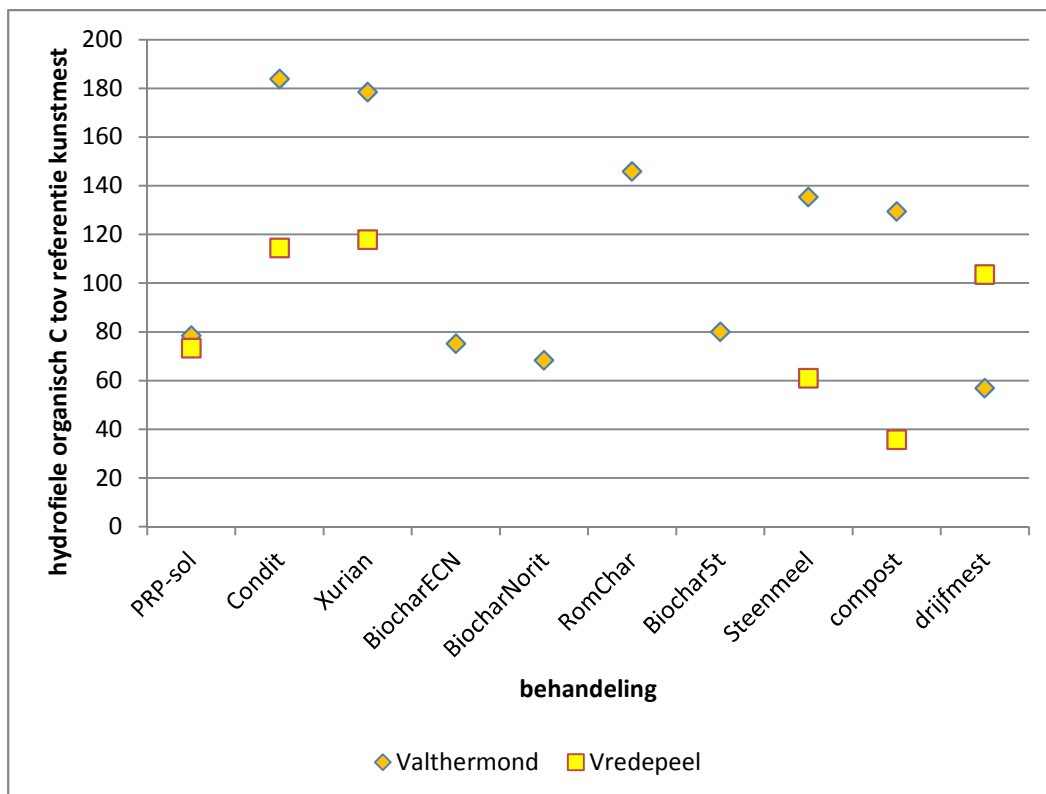
Figuur 4.23 De hydrofiële organische stof op de twee zandlocaties. De waarde op de referentieobjecten te Valthermond en Vredepeel bedroeg respectievelijk 1,14 en 1,70, mg C /l.
