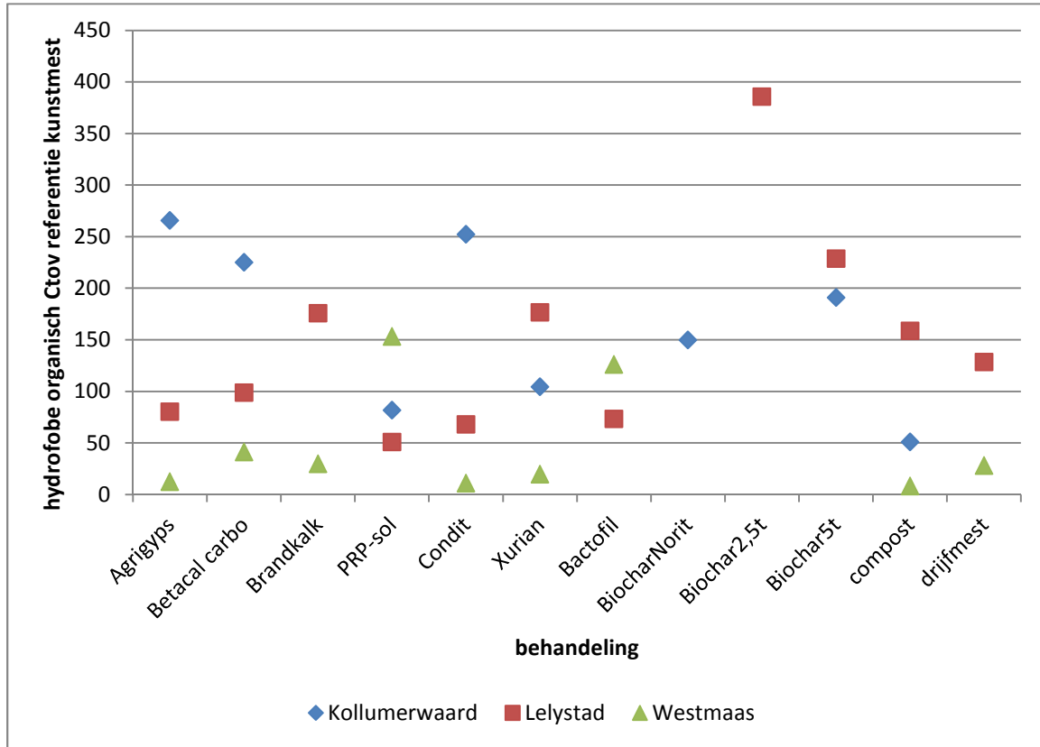
Figuur 4.20 De hydrofobe organische stof op de drie kleilocatie. De waarden op de referentieobjecten in Kollumerwaard, Lelystad en Westmaas bedroegen respectievelijk 0,85, 1,22 en 7,13 mg C /l. NB: Brandkalk en drijfmest in Kollumerwaard bedroegen 975 en 781 mg C /l.
