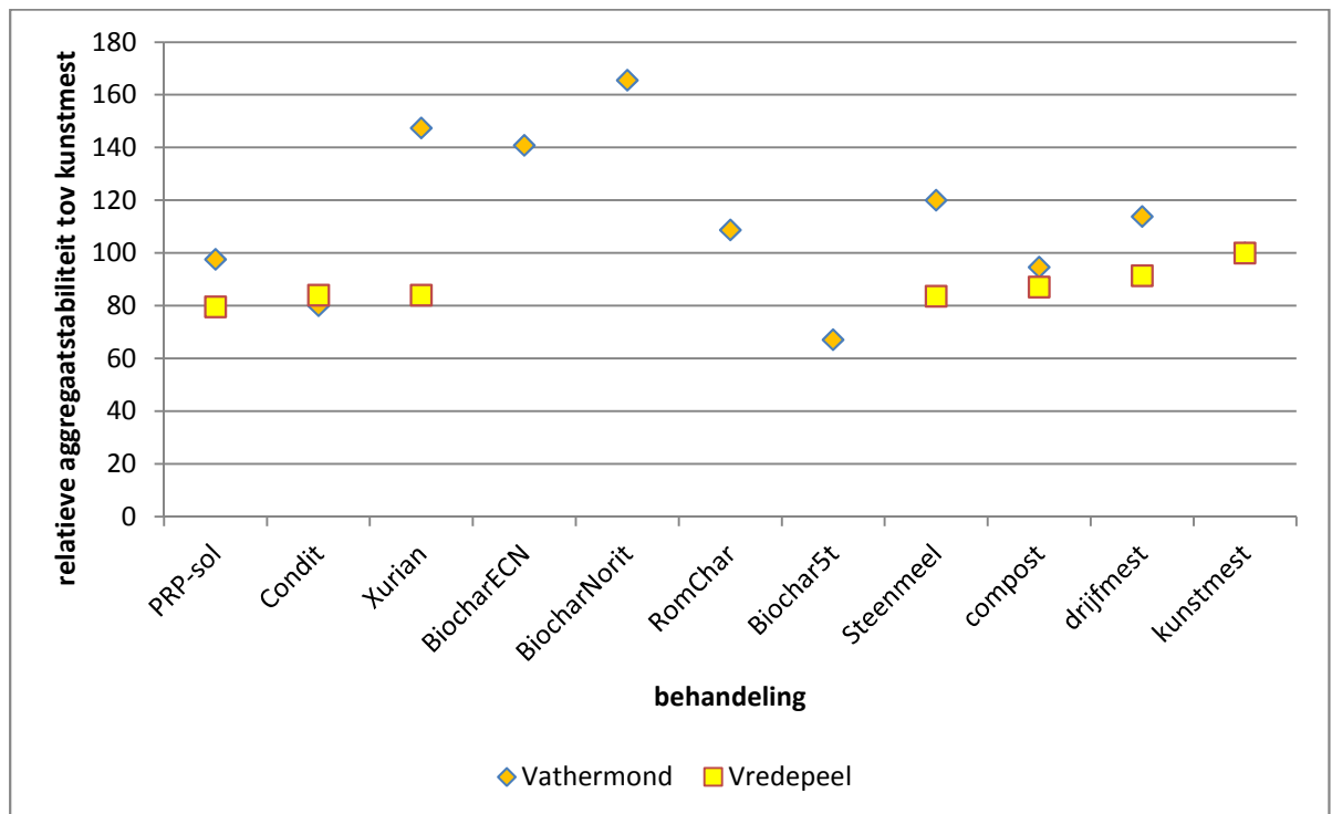
Figuur 4.6 De relatieve aggregaatstabiliteit-index op de twee zandlocaties ten opzichte van kunstmest (referentie kunstmest: Valthermond=0,19, Vredepeel=0,61), %.
