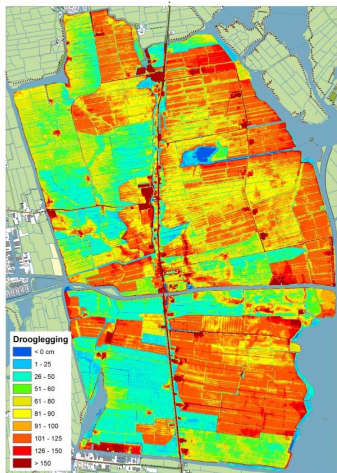
Figuur 6.9 Drooglegging in de zomer (cm)
