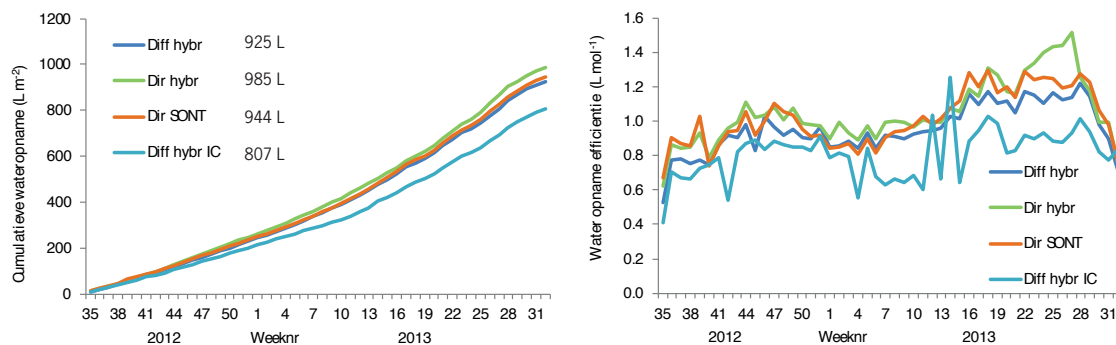
Figuur 25. Cumulatieve wateropname ( L \cdot m^{-2} ) tijdens de teelt links. Rechts de efficiëntie van wateropname in liters per mol licht ( L \cdot mol^{-1} ) gedurende de teelt.
