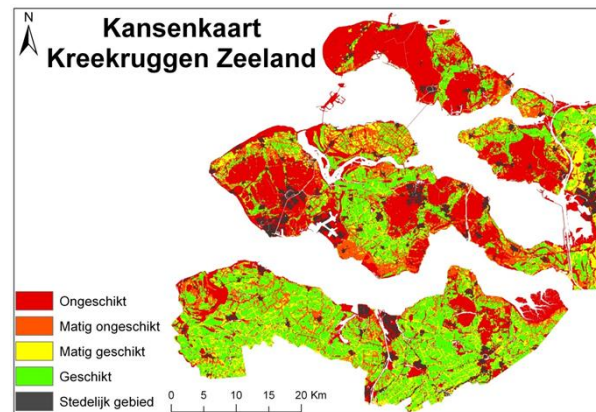
Fig. 18: kansenskaart voor opschaling van de Kreekrug Infiltratie Proef. Detail metingen zijn nodig voor een verdere analyse.
