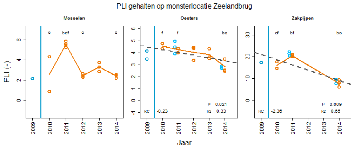
Figuur 1: Trend in metaalgehalten (PLI) in mosselen ( Mytilus edulis ), oesters ( Crassostrea gigas ) en zakpijpen ( Ciona intestinalis ) op de Zeelandbrugpijler van 2009 tot en met 2014. Donker blauwe datapunten geven T0 bemonstering weer, verticale lijn scheidt jaren voor en na stort van oeververdediging. Licht blauwe punten betreffen metingen op de referentielocatie Zuidbout.
