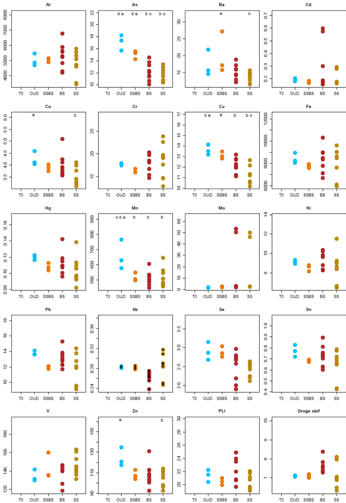
Figuur 23: Metaalgehalten, PLI en drogestof in Ciona intestinalis bemonsterd op verschillende ondergronden bij de Zeelandbrug in 2011. De ondergrondtypen worden als volgt aangeduid: T0 = meting voor bestorting, OUD= oude ondergrond op referentielocatie, BS = breukstenen, SS = staalslakken, SSBS = staan onder invloed van staalslakken en breukstenen. Metaalgehalten die onder de detectielimiet liggen worden weergegeven met zwarte stippen. De lettercode geeft significante verschillen weer (ANOVA, Tukey Posthoc).
