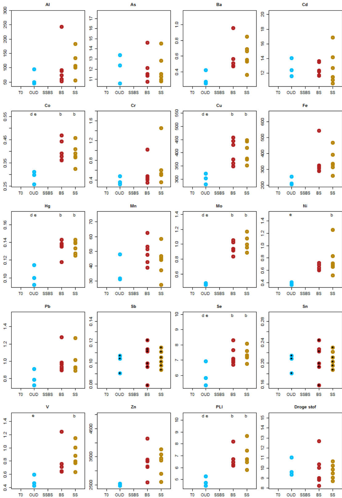
Figuur 33: Metaalgehalten, PLI en drogestof in Crassostrea gigas bemonsterd op verschillende ondergronden bij de Hoedekeskerke in 2014. De ondergrondtypen worden als volgt aangeduid: T0 = meting voor bestorting, OUD= oude ondergrond op referentielocatie, BS = breukstenen, SS = staalslakken, SSBS = staan onder invloed van staalslakken en breukstenen. Metaalgehalten die onder de detectielimiet liggen worden weergegeven met zwarte stippen. De lettercode geeft significante verschillen weer (ANOVA, Tukey Posthoc).
