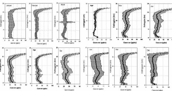
Gambar 2. Rata-rata bulanan profil vertikal ozon Watukosek (1993-2005) serta standar deviasinya untuk bulan Januari sampai Desember
