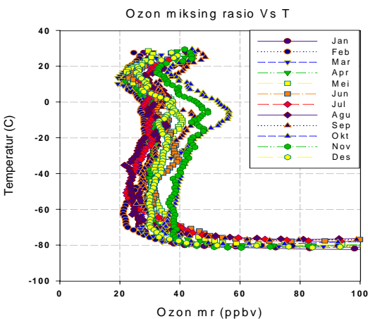
Gambar 6. Korelasi ozon miksing ratio dengan Temperatur
