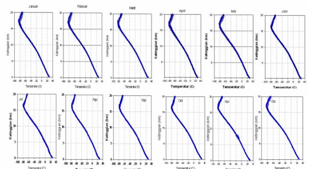
Gambar 4. Rata-rata bulanan profil vertikal temperatur Watukosek (1993-2005) serta standar deviasinya Januari – Desember
