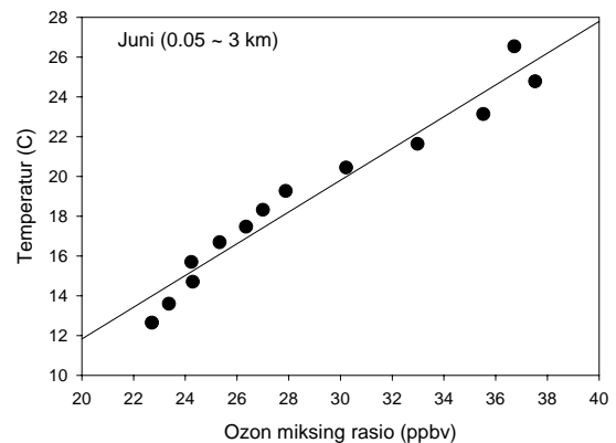
Gambar 7. Contoh plot korelasi temperatur dan ozon bulan Juni pada ketinggian 0.05 – 3 km
