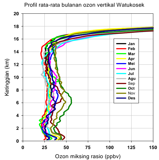
Gambar 3. Rata-rata bulanan profil vertikal ozon Watukosek bulan Januari sampai Desember.
