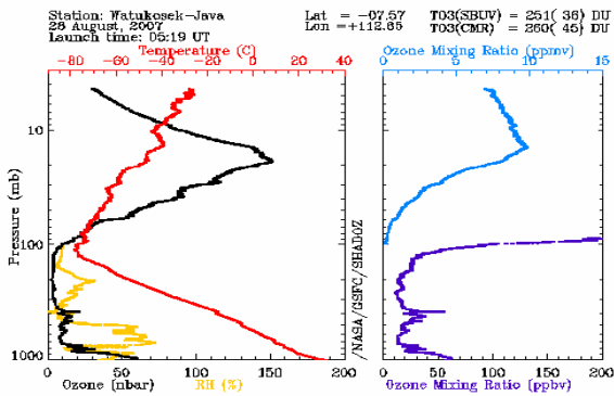
Gambar 1. Contoh profil ozon, temperatur dan kelembaban (kiri) dan ozon miksing rasio (kanan) Watukosek yang dipublikasi di web-NASA
