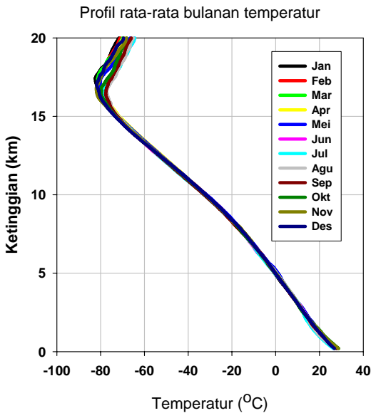
Gambar 5. Rata-rata bulanan profil vertikal temperatur Watukosek Januari – Desember
