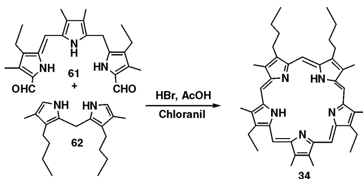
Scheme 17.
