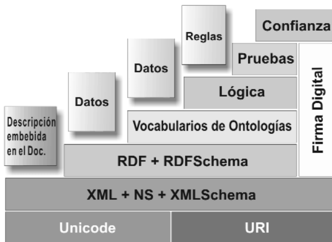
Semantic Web "layer cake" (Berners-Lee. XML Conference, 2002)
