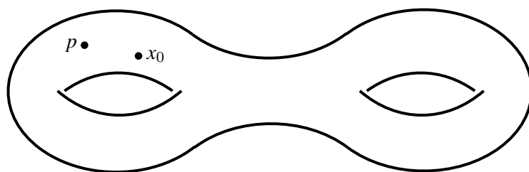
Figura 4.2: Superficie de género 2 con un punto singular de orden 3.
