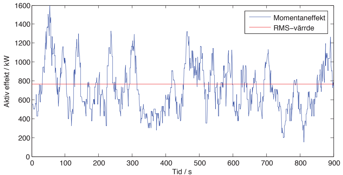
Figur 20 - Aktiv effekt på sekundärsidan av T17
