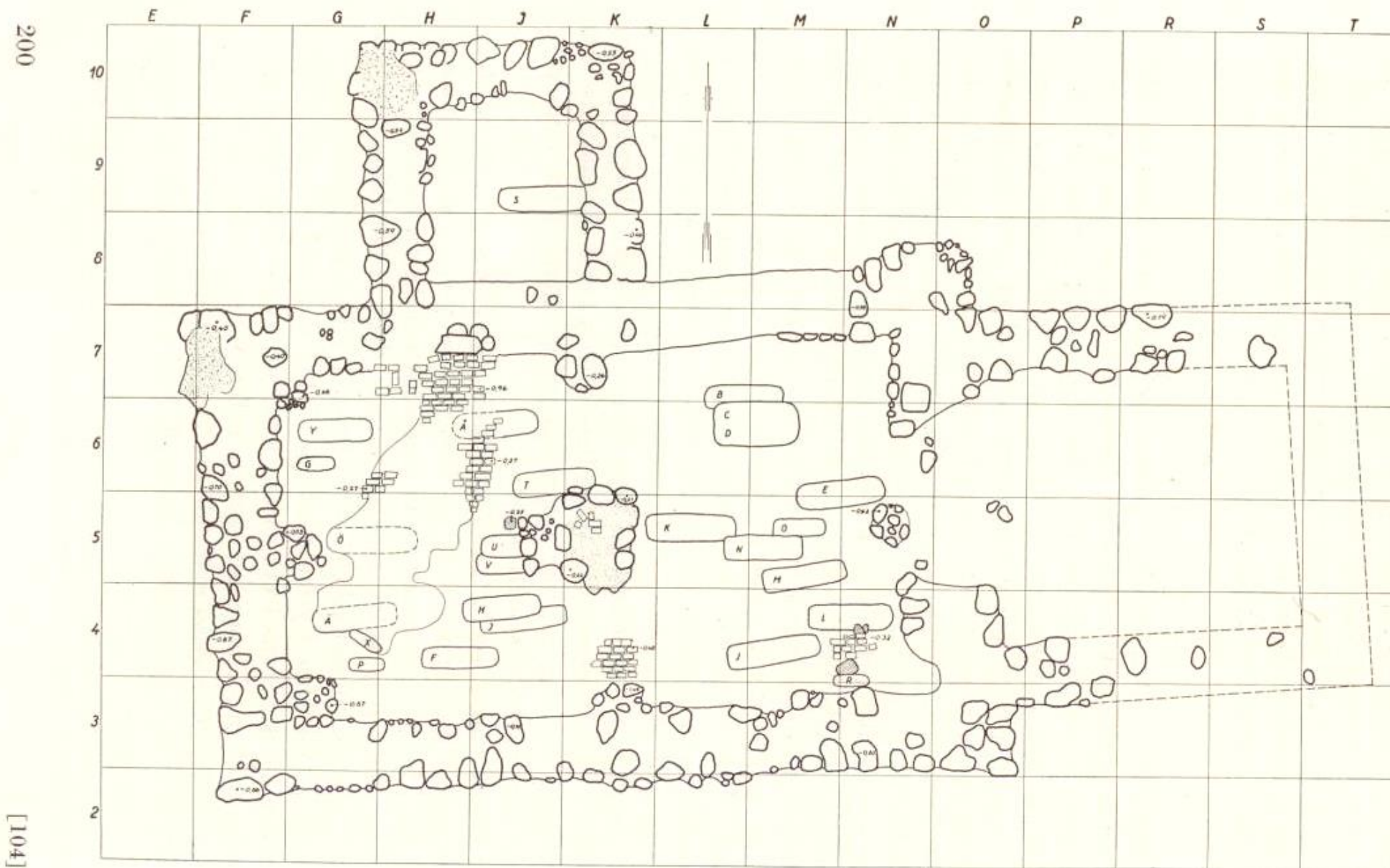
Fig. 3. Plan över kyrkan med inlagda gravar.
