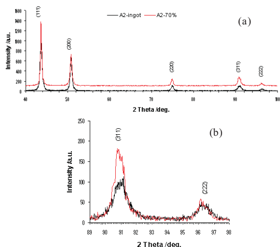
Gambar 4. Pola difraksi spesimen baja 15%Cr-25%Ni; (a). full profile dan (b). pergeseran puncak bidang (311) dan (222) pada ingot as cast dan rol panas 70% reduksi ketebalan.
