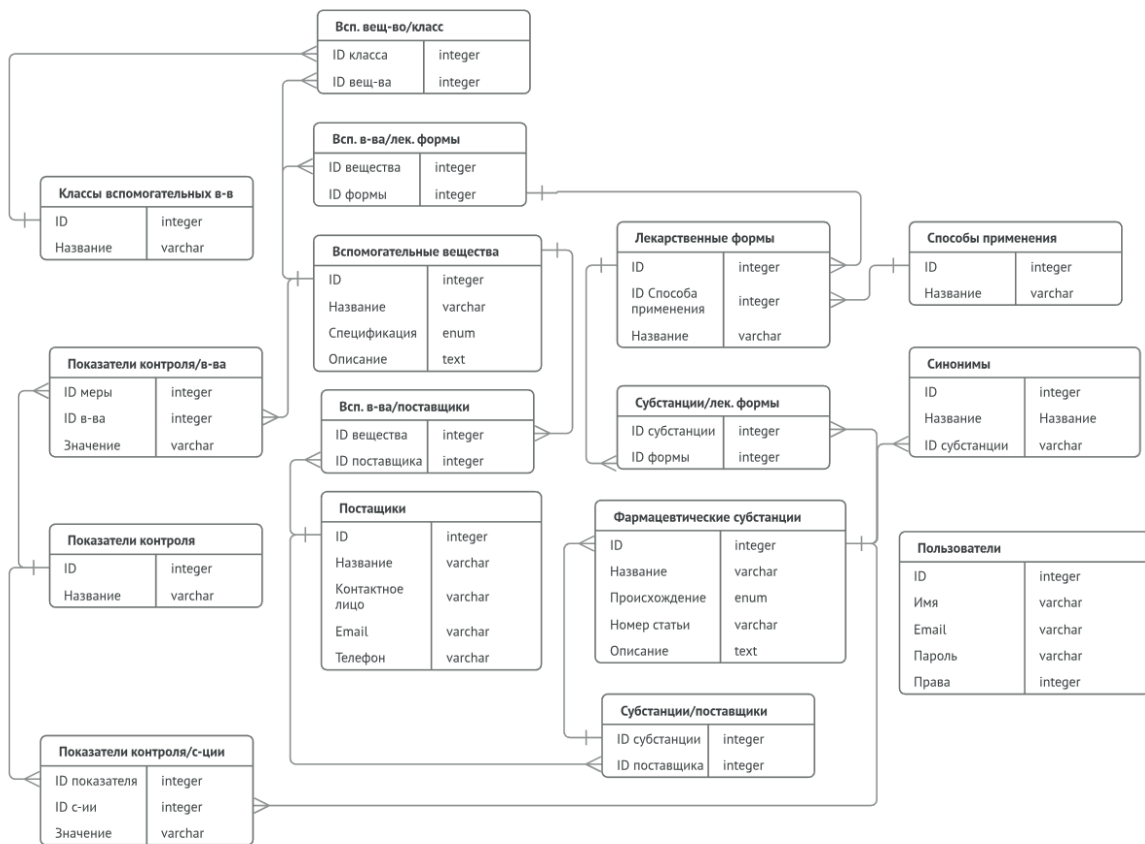
Рис. 6. Реляционная модель данных базы данных лекарственных и вспомогательных веществ.
