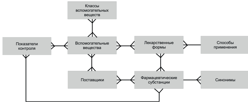
Рис. 5. Модель «Сущность-связь».
