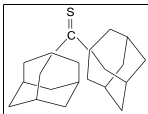
Figure 27. Structure of bis -(1-adamantyl) thioketone.
