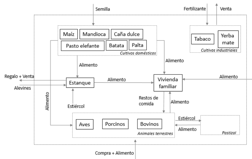
Figura 4.10. Diagrama de flujo de la explotación modelo 3.
