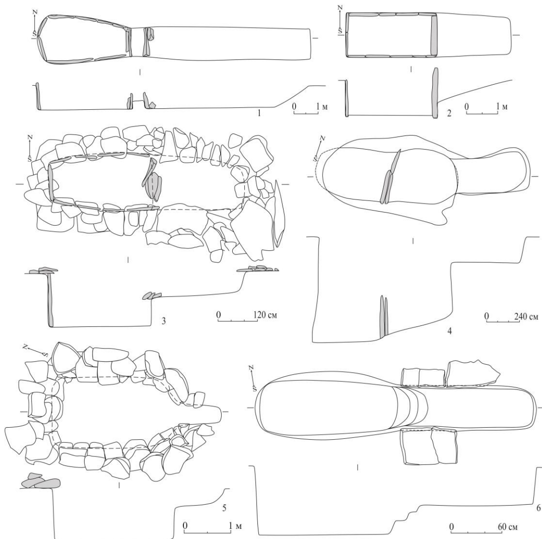
Рис. 3. Типы дромосных могил: 1 – курган 1 могильника Талды-2; 2 – курган с «усами» Назар; 3 – курган 12 могильника Бақыбулак; 4 – курган 10 могильника Серекты-1; 5 – курган 9 могильника Карашоқы; 6 – курган 1 могильника Шерубай
