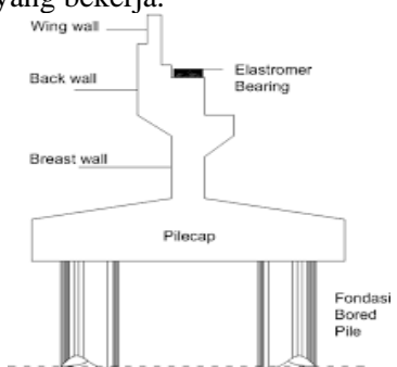
Gambar 1. Bagian-bagian Pada Abutment
