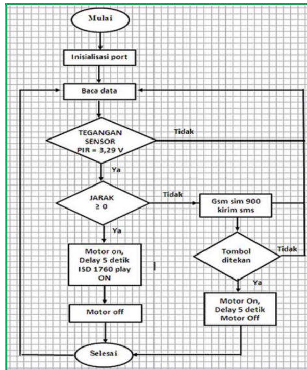
Gambar 8. Flowcart Sistem Tempat Sampah Otomatis
