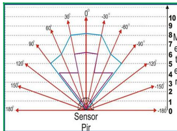
Gambar 10. Jangkauan Sensor PIR Pendeteksi Kedatangan Orang
