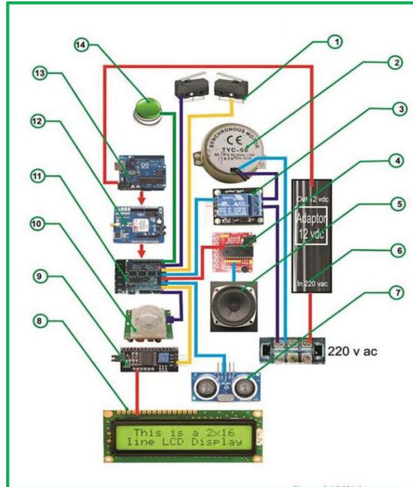
Gambar 3.2 Blok Diagram Komponen Tempat Sampah Otomatis
