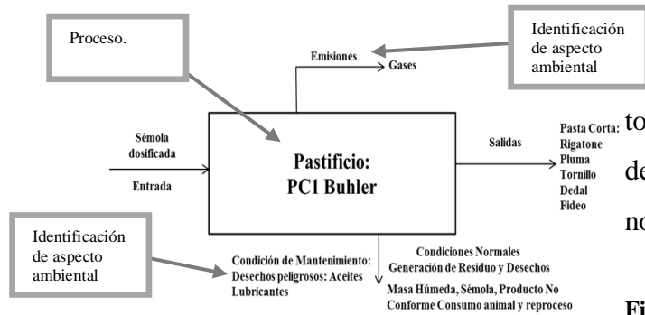
Figura 2. Identificación de aspectos ambientales en el proceso productivo de la línea de Pastas Corta 1 PCI Equipo Buhler.
